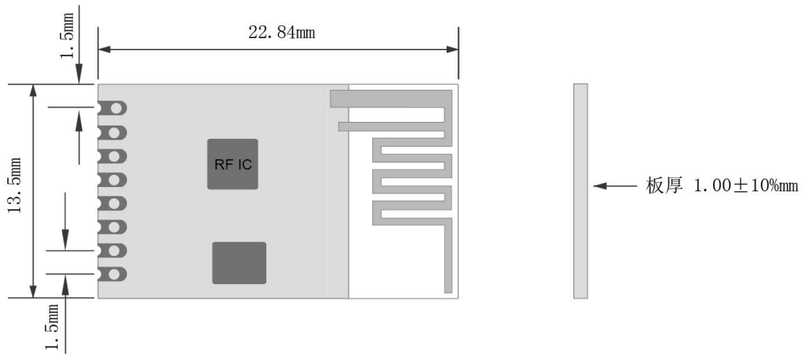
DL-297LDA-S 尺寸图
