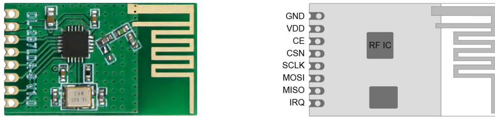
DL-297LDA-S 系列引脚定义
