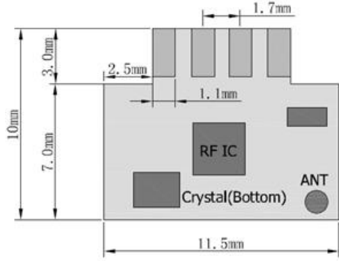
DL-297LD 尺寸图
