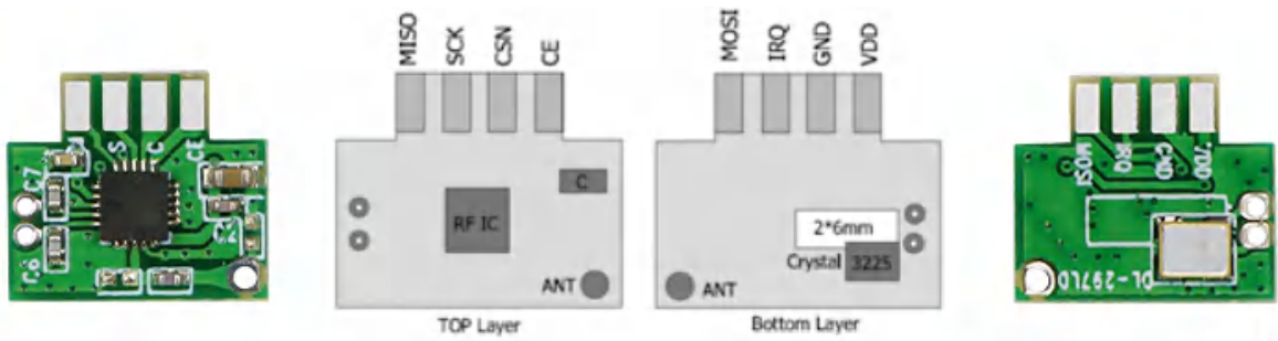
DL-297LD/ DL-297LDA 引脚定义
